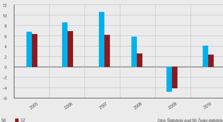
Graf 1 Reálny medziročný rast HDP v lokálnej mene
